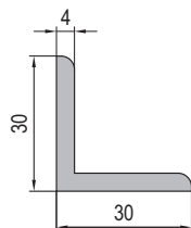
Angle Profile 30x30x4 角铝型材 30x30x4
