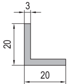
Angle Profile 20x20x3 角铝型材 20x20x3
